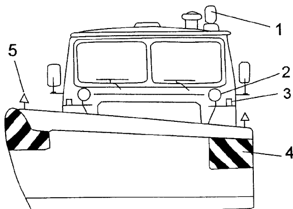
Rys. 3. Oznakowanie pluga i nośnika 1 – lampa ostrzegawcza barwy żółtej, 2 – reflektory samochodu podniesione na wspornikach, 3 – kierunkowskazy umieszczone na wspornikach, 4 – biało-czerwone odbłaskowe pasy na końcach odkładnicy, 5 – lampa biała widoczna z przodu i czerwona widoczna z tyłu
